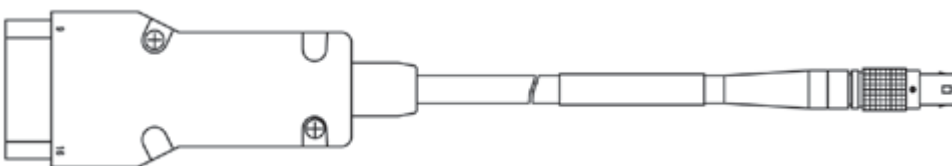
CAN インターフェースケーブル、OBDII J1962 - Lemo 1B FGC (16mc-8mc)、2m50
