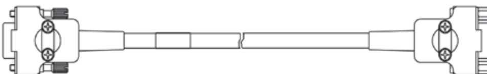
Câble d'interface CAN, FlexRay et LIN en Y, Lemo 1B FGC - 2xSUB-D (8mc-9fc+9mc), 2 m
